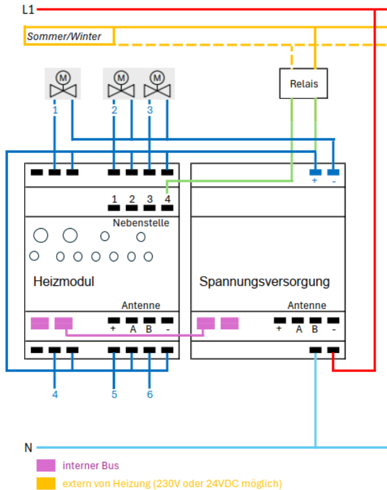
Variante 24VDC
