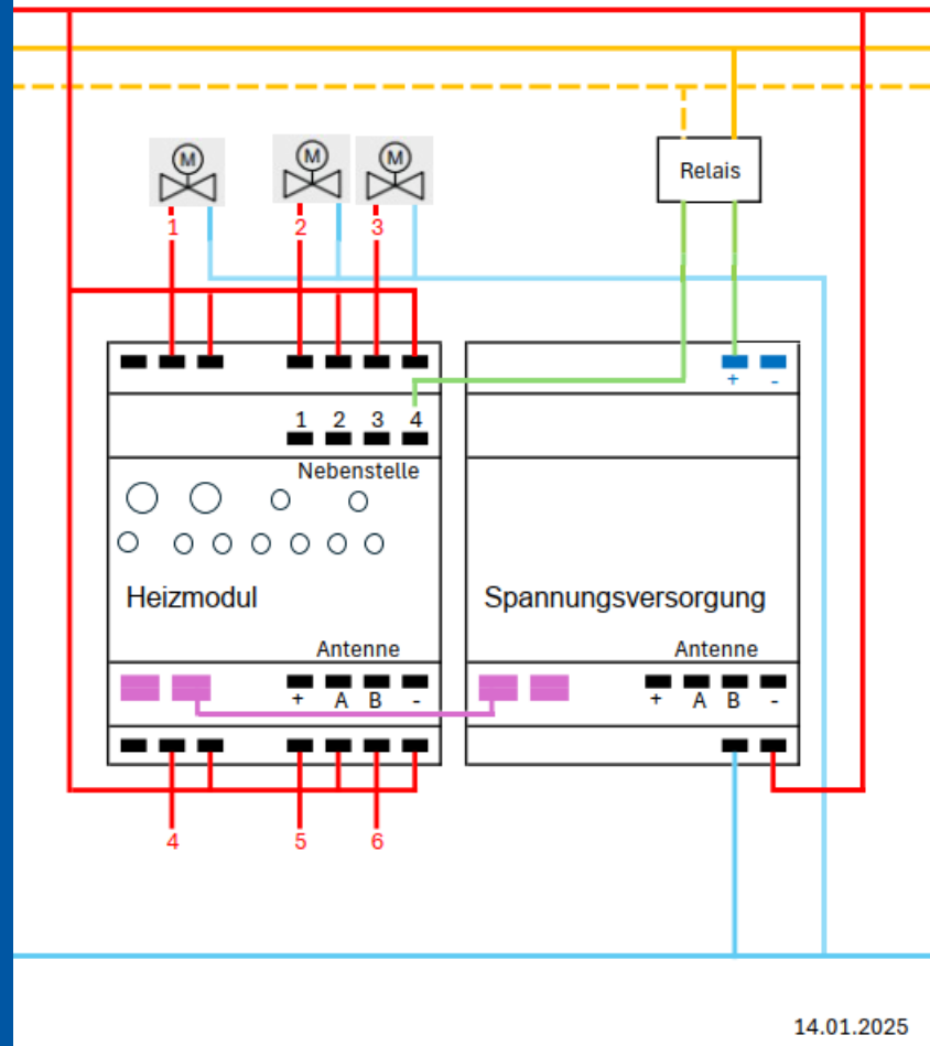
Variante 230V
